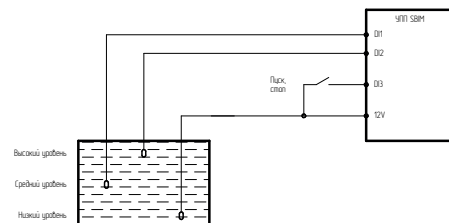
Датчик уровня 3
