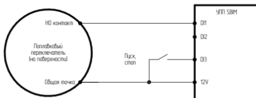
Датчик уровня 3
